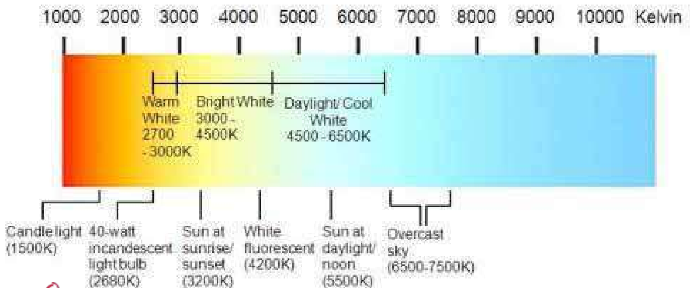
شكل (٣) وحدات Kelvin و علاقتها بالطول الموجي للضوء
