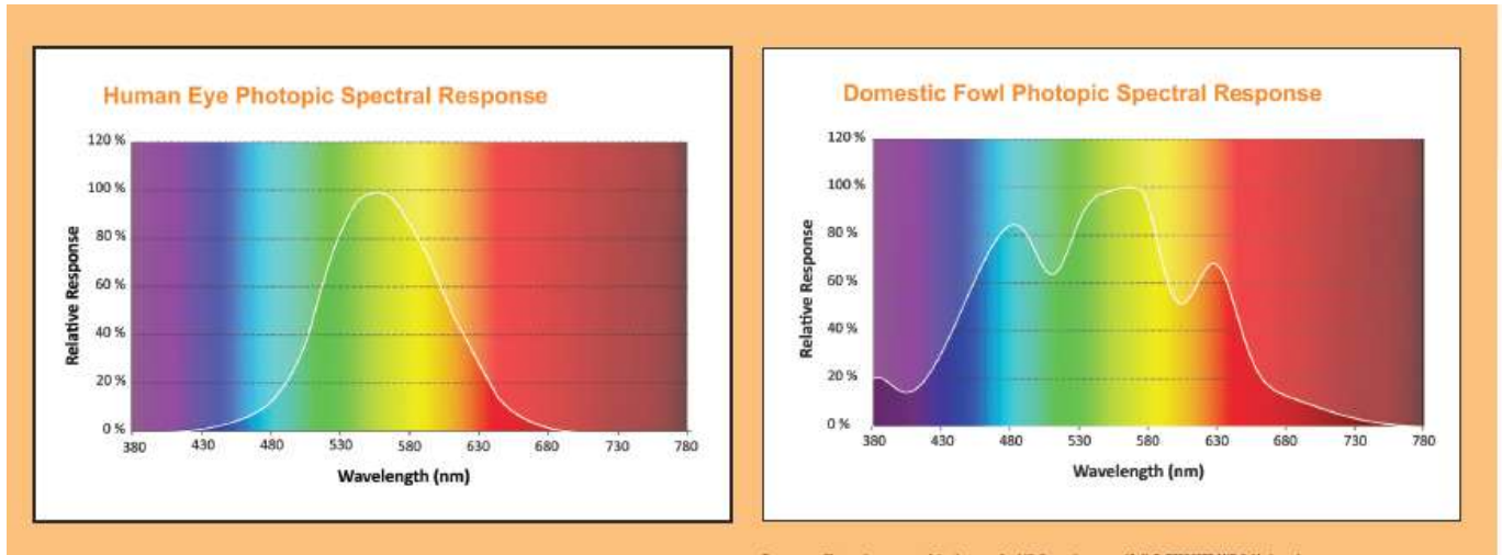
شكل (٢) استجابة الطيور الداجنة و الانسان للطول الموجي للضوء
