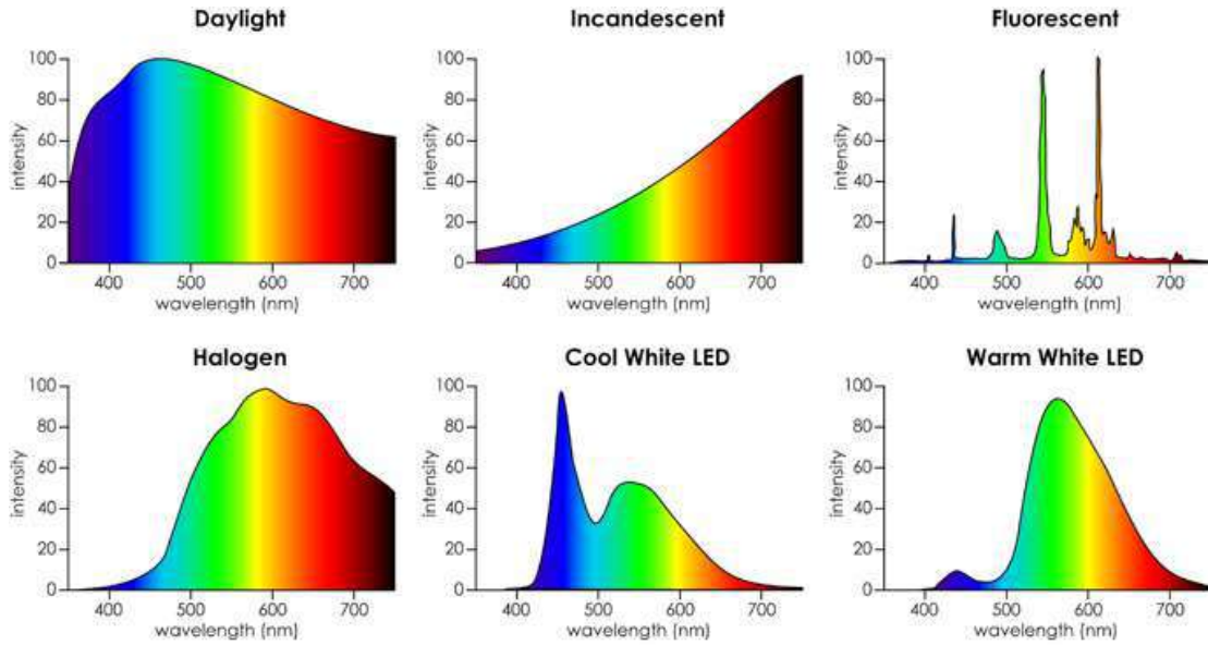
شكل (٤) التحليل الطيفي للضوء الصادر عن أنواع اللمبات المختلفة
